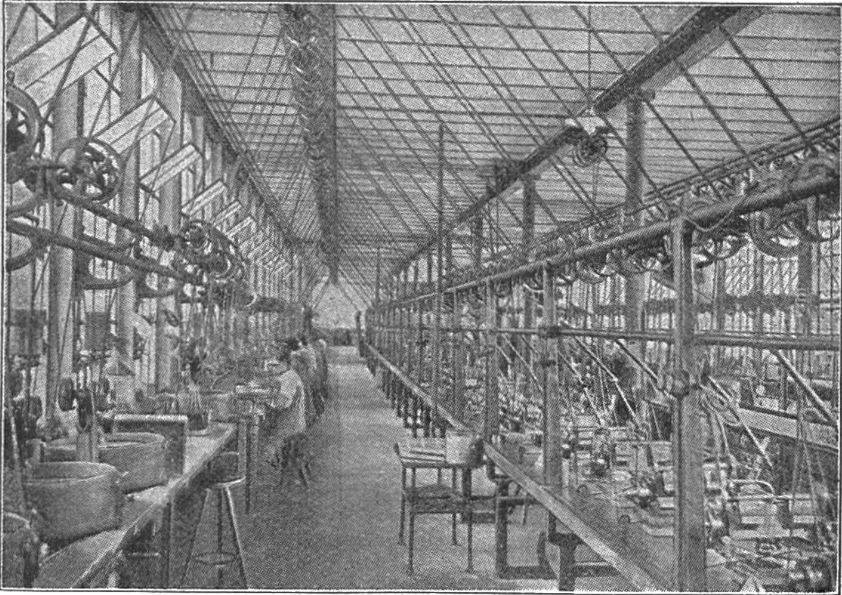
Teilansicht eines Arbeitsraumes „Zenith“ für Stahlstücke.
