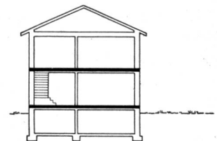
BRUTTO - WOHNFLÄCHE = FLÄCHE DER BEWOHNTEN GESCHOSSE INCL. MAUER - KORRIDOR- U. TREPPEN- HAUSFLÄCHEN = GEBÄUDEGRUNDFLÄCHE MAL ZAHL DER GESCHOSSE
