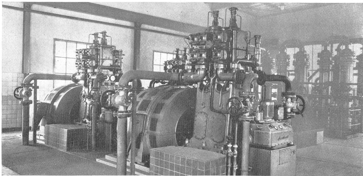
Kompressorstation der Gasfernleitung Saarbrücken-Paris
