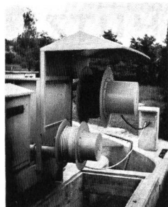
Federkabeltrommel als Längsstromzuführung an einem Längsräumler in einer Kläranlage, Kabelabzug horizontal
