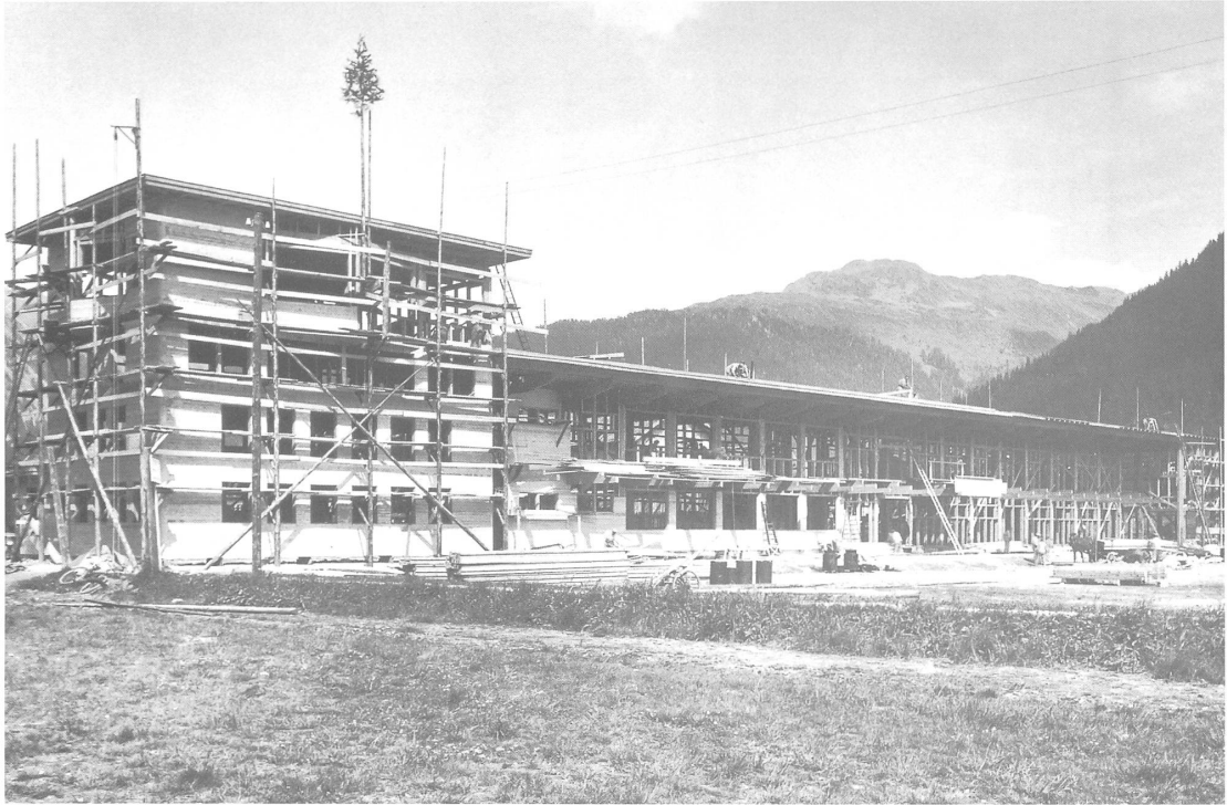
Abb. 4: Eisbahngebäude Davos. Aufgerichteter Rohbau
