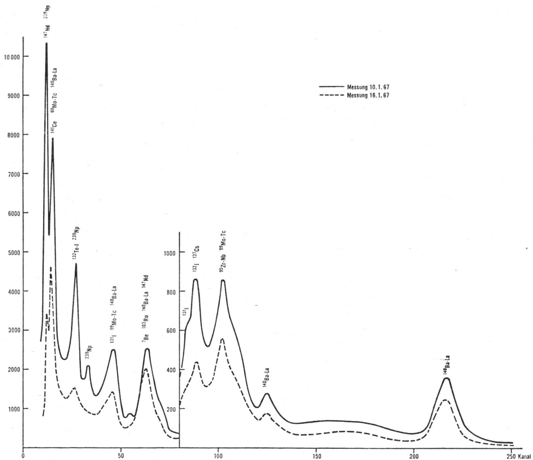
Fig. 4. Gammasppektrum eines Luftfilters aus 8400 m Höhe (obere Troposphäre), gesammelt am 9.1.67, gemessen am 10. und 16.1.67.
