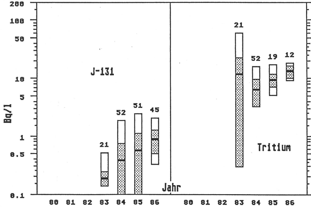
Fig.4.4.c: ARA Basel
