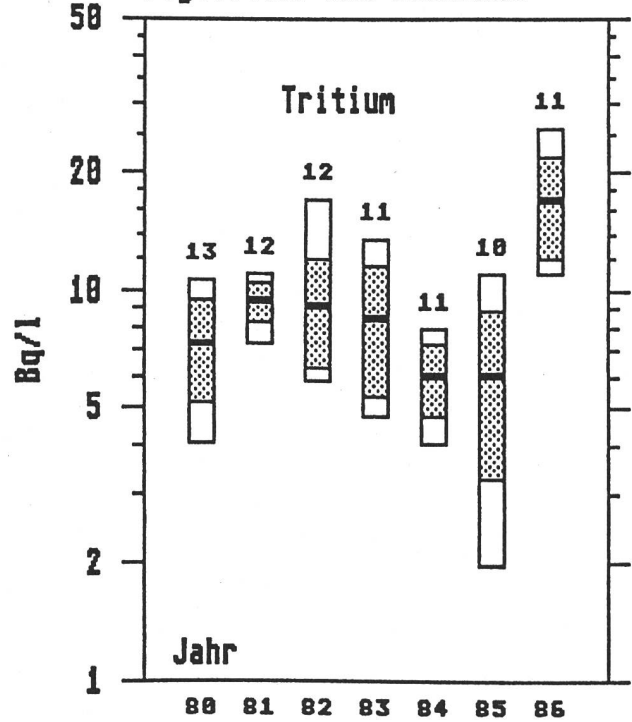
Fig.4.4.e: ARA Lausanne
