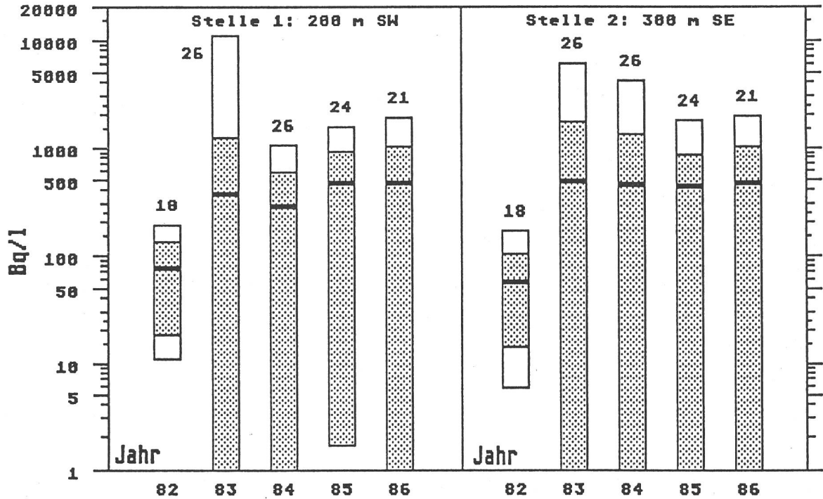
Fig.4.2.b: Tritium im Niederschlag Umgebung MB Microtec, Niederwangen/BE
