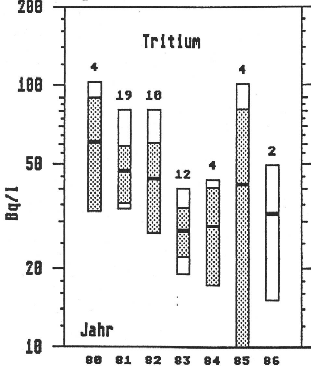
Fig.4.4.d: ARA Teufen
