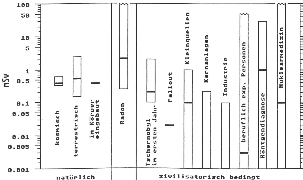
Fig.7.1.b: Zusammenfassung der Strahlendosen (logarithmisch) (effektive Äquivalentdosis pro Jahr)
