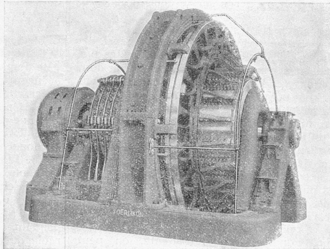
COMMUTATRICE 5000 KW, 10.000 AMPÈRES
