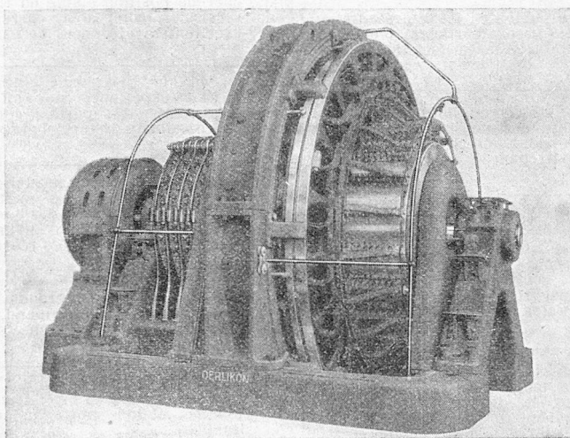
COMMUTATRICE 8000 KW. 10.000 AMPÈRES
