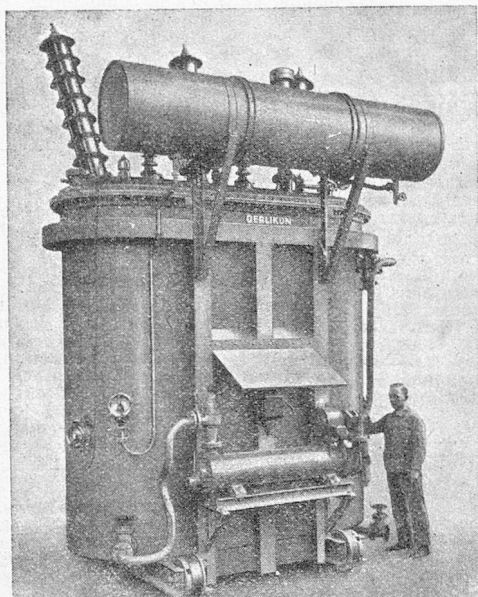
TRANSFORMATEUR POUR EXTÉRIEURS 3000 KVA 11500/23500 V DTS AVEC CONSERVATEUR ET RÉFRIGÉRANT
