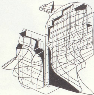
Cartographie du rayonnement acoustique d'un moteur thermique
