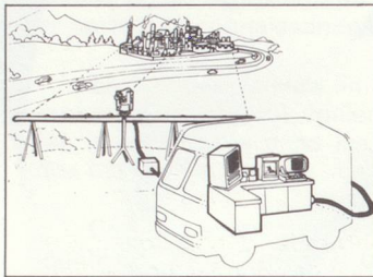
Analyse acoustique de sites bruyants en champ lointain.
