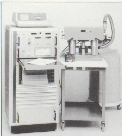
Viscoélasticimètre : mesure des caractéristiques dynamiques des matériaux viscoélastiques.
