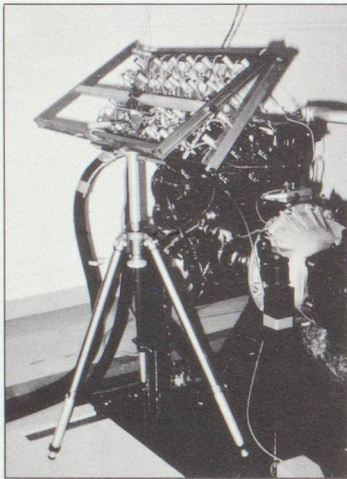
Cartographie du rayonnement acoustique d'un moteur thermique
