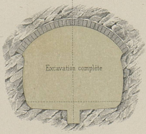
Profil achevé avec voûte. (pas encore exécuté)
