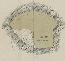
Profil en a.
