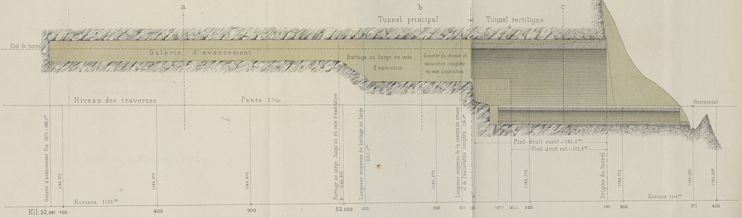
Profil avec revêtement complet. (pas encore exécuté)
