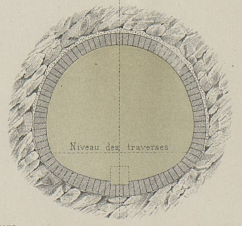
Profil avec revêtement complet. (pas encore exécuté)
