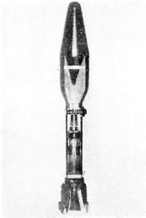
Razzo anticarro « Bazooka » usato dall'Aviazione Americana (capacità di perforazione: corazza d'acciaio di 28 cm.).
