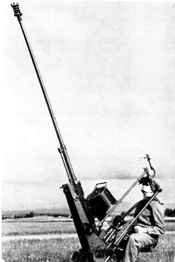
Svizzera: Cannone di DAA del tipo 6 ILa/5 TG; calibro 20 mm.- Velocità di tiro 1000 colpi al minuto
