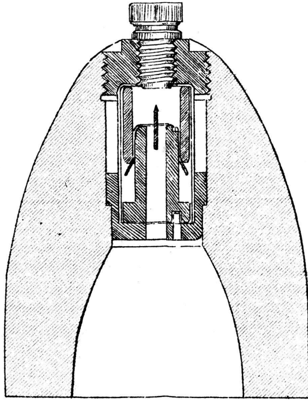
Godet de suspension en acier.
