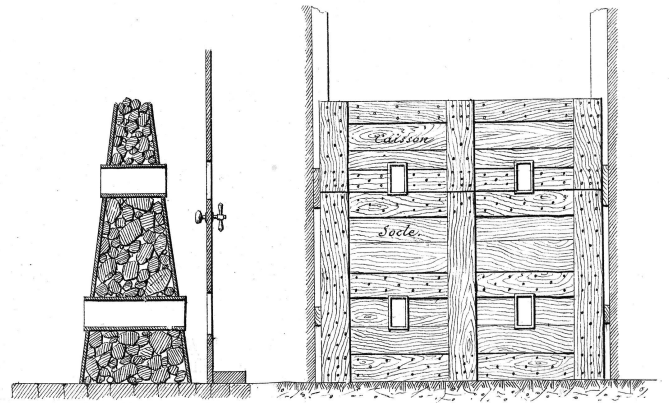
Fig. 14. Echelle 1/10.
