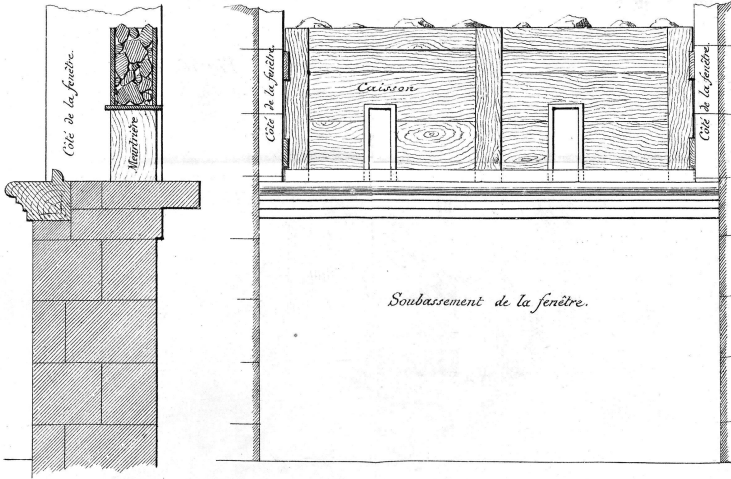
Fig. 13 Profil Echelle 1/10.
