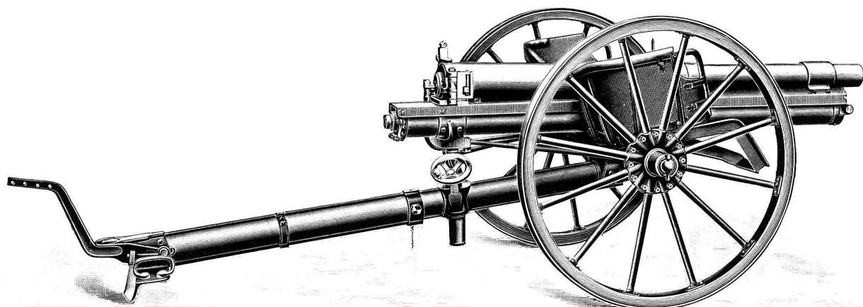
Canon Ehrhardt à tir rapide c/1900 ( flèche raccourcie ).
