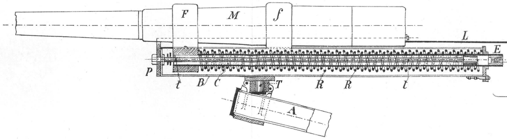
fig. 1. Bouche à feu et berceau.
