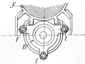
fig. 4 Vue arrière du berceau.
