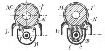
fig. 3 Coupe suivant f fig. 2 Coupe suivant F.
