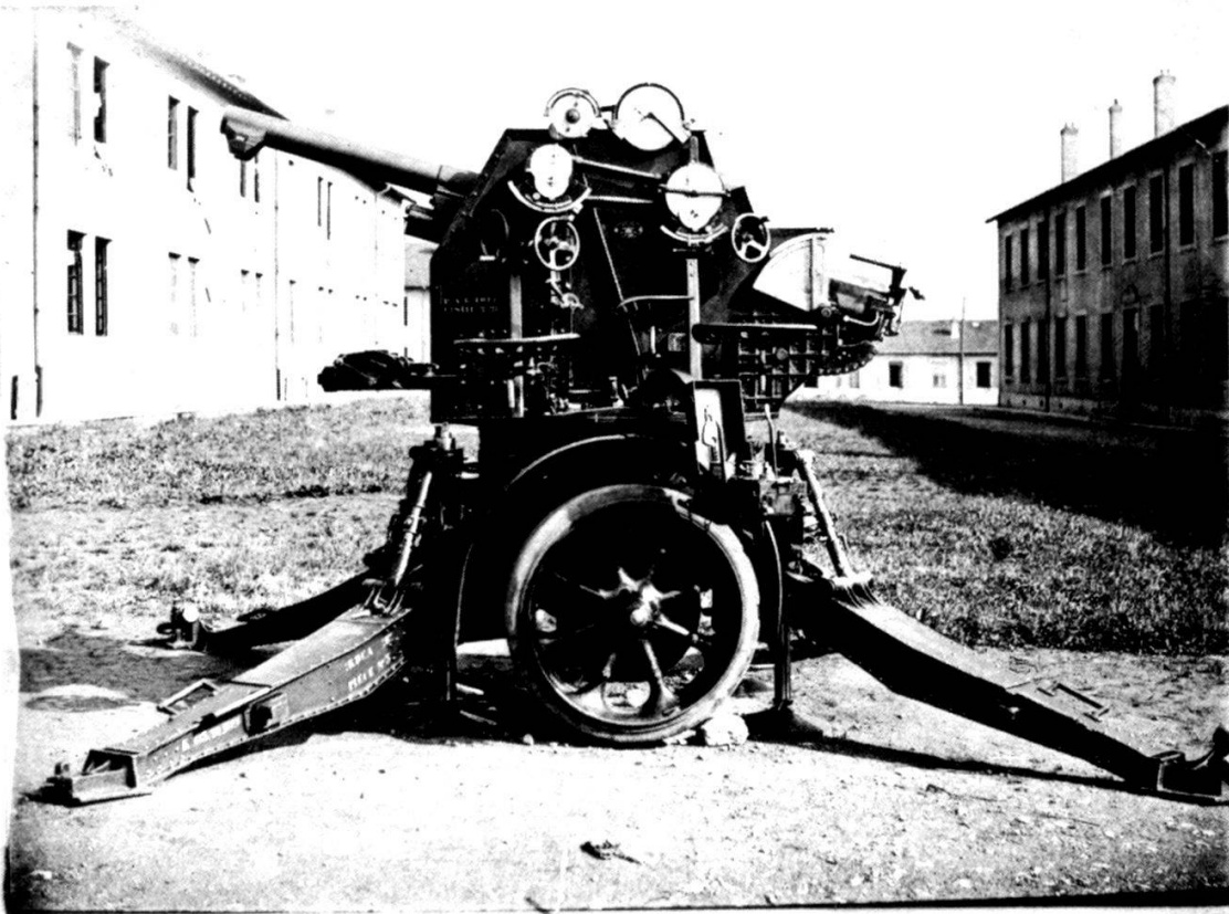
Canon de 75 mm contre avions, portée 5000 mètres. 8 servants. (Photo A. Wingerter prise en 1931 au 403 e Rgt de DCA à Toul.
