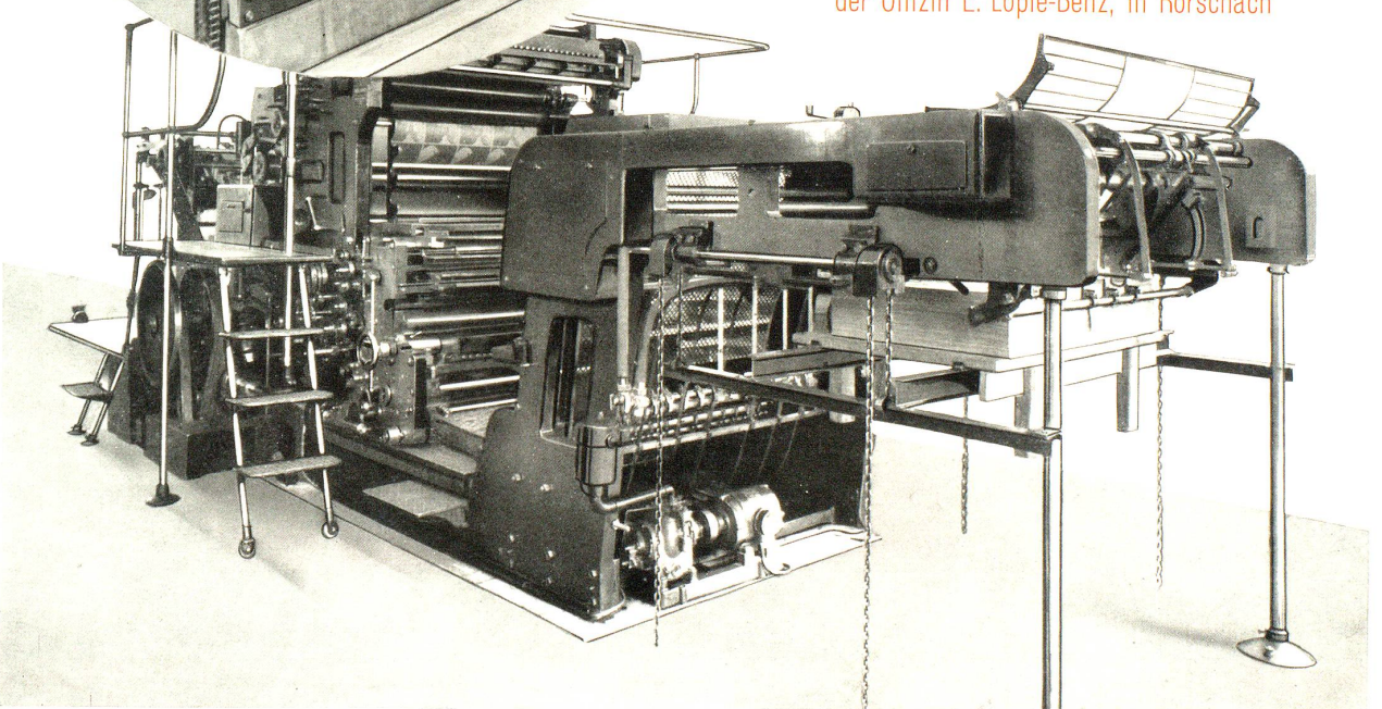
Die Ein- und Mehrfarben-Offset-Druckmaschinen der Offizin E. Löpfe-Benz, in Rorschach
