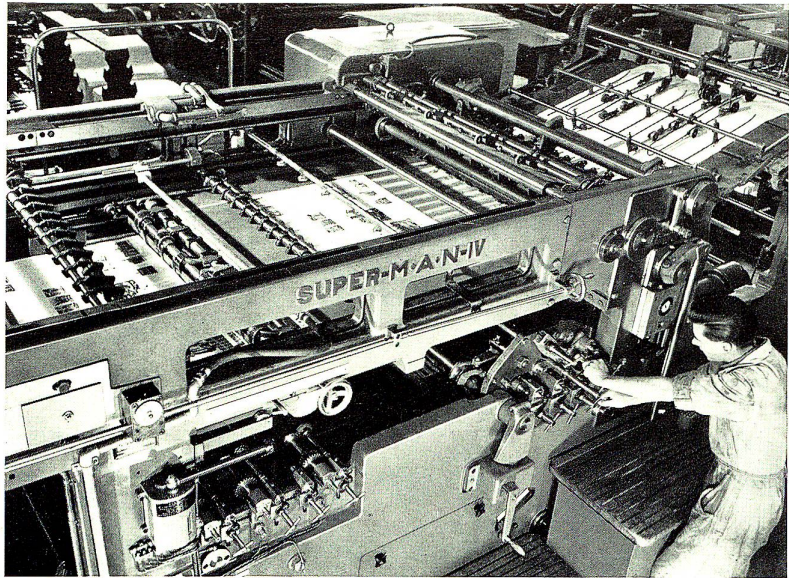
Super MAN IV Zweitouren-Buchdruckmaschine
