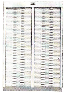
KT 192: 192 Auszüge für unmontierte Klischees. Schrank: 1000x675x675 mm Schieber: 7x270x520 mm Nutzfläche 27 m 2
