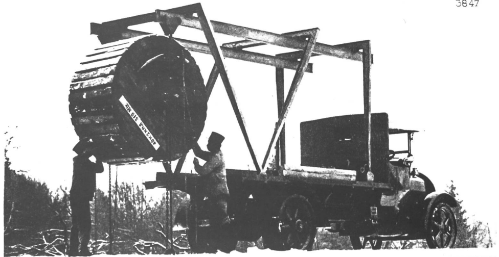
CAMION 5 TONNES AVEC DISPOSITIF DE CHARGEMENT 5 TONNEN LASTWAGEN MIT LADERVORRICHTUNG 5 TON LORRY WITH LOADING APPARATUS
