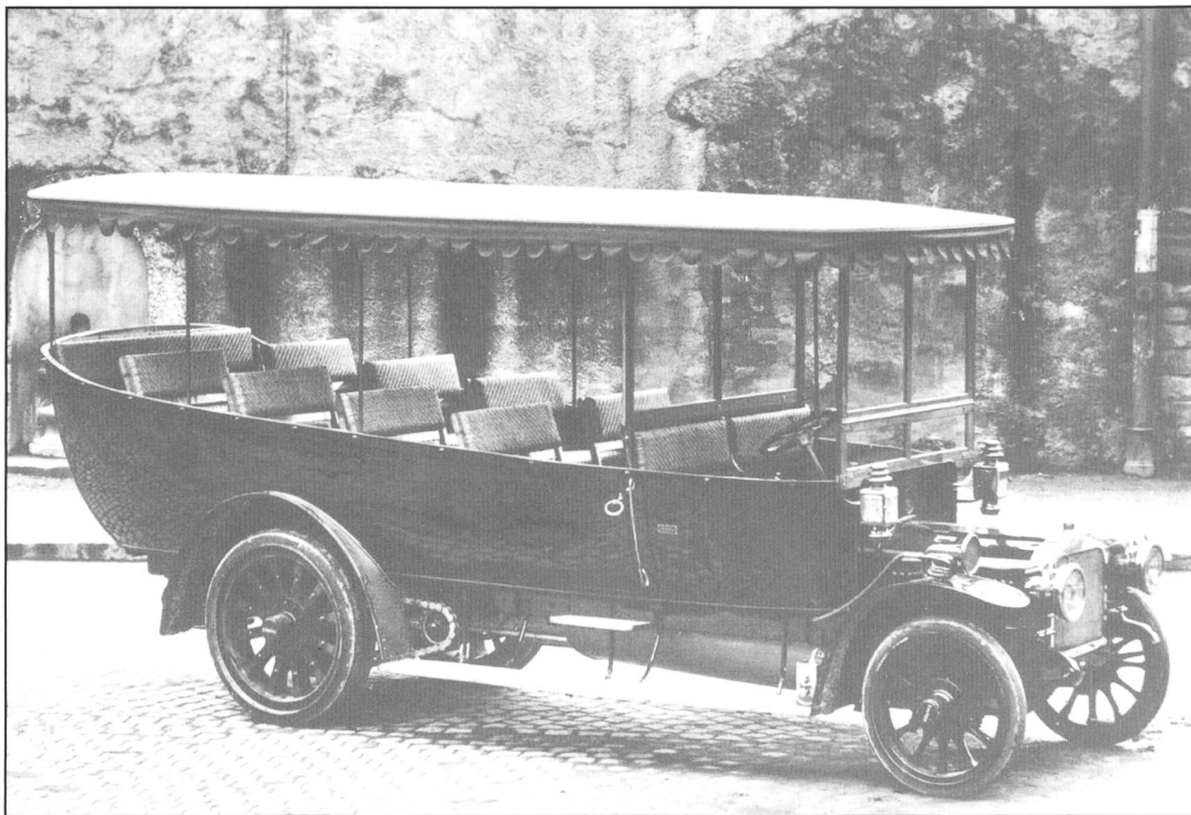
Auto Avienda, 3 Tonnen-Kettenwagen für Personenbeförderung, 1910
