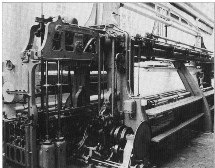
lochkartengesteuerte-Schiffli-Stickmaschine
