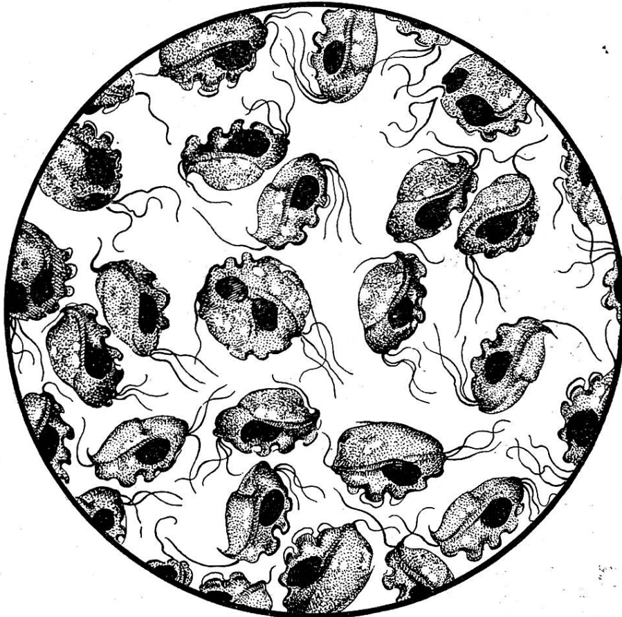
Trichomonas foetus
