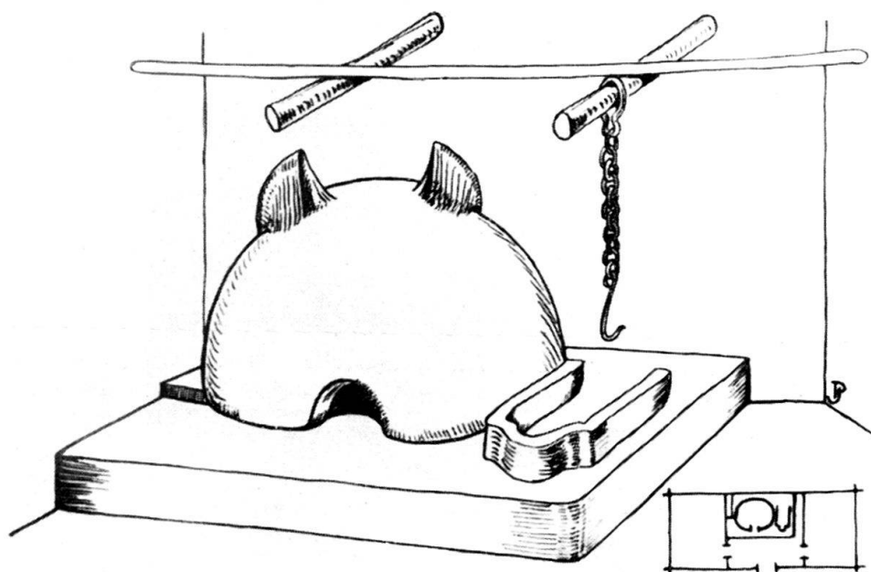
Abb. 2. Ofen mit Lehmohren. Dorf Torockószentgyörgy, Siebenbürgen.
