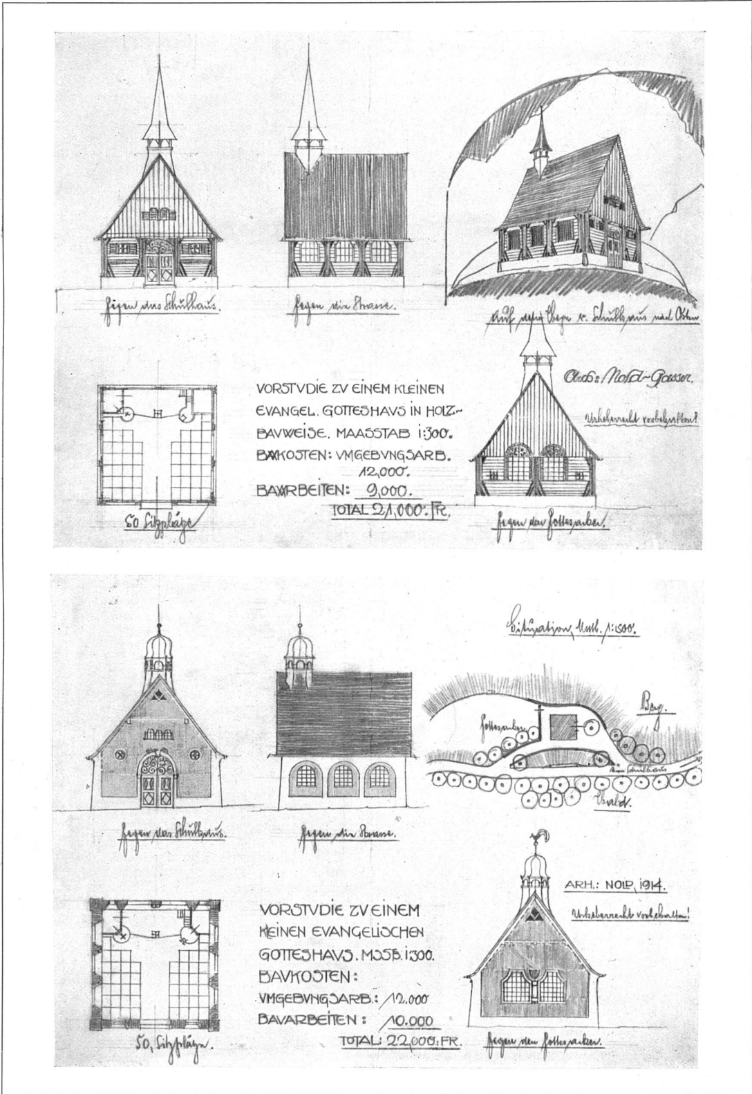
Zwei Vorstudien zu einer kleinen evangelischen Kapelle im Gebirge. Architekt Nold, Felsberg bei Chur.
