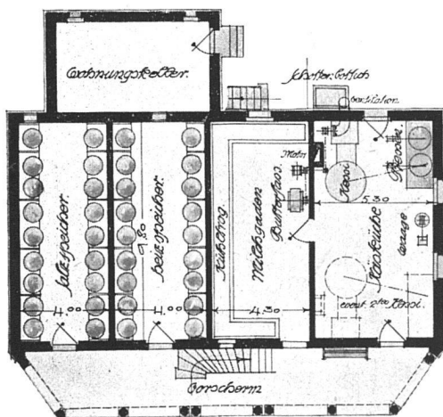
Erdgeschoß. Käseerei Vinelz (Seeland). — Grundrisse.
