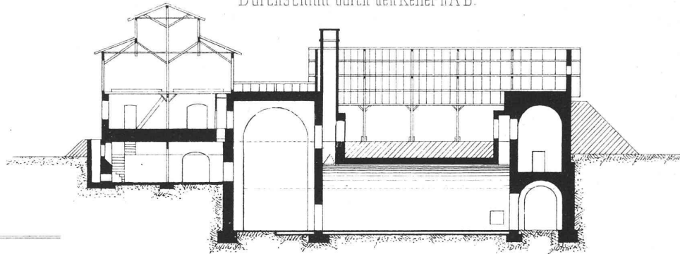
Durchschnitt durch den Keller nA B.
