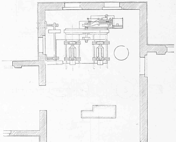
Masstab 1 : 100.
