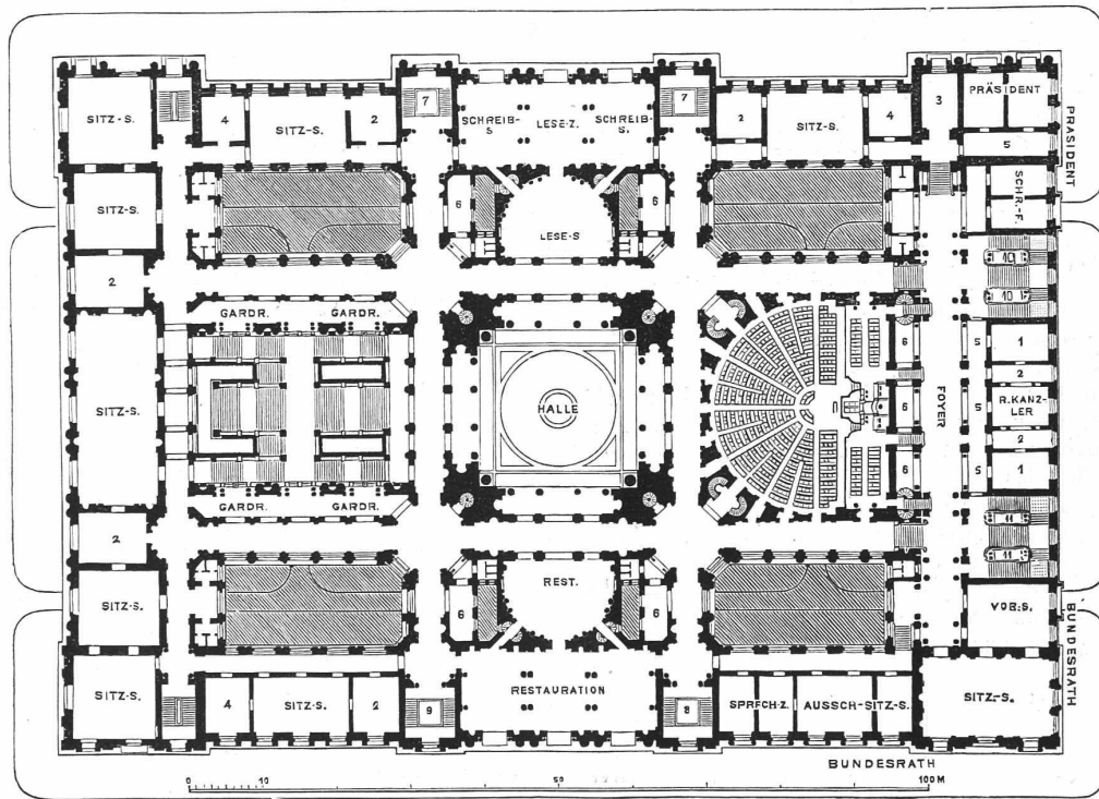
Grundriss des Hauptgeschosses.
