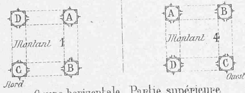
Coupe horizontale - Partie supérieure
