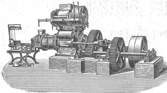
Grosse Ziegelmachine mit Walzwerk.
