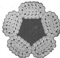
Patentiert „flachlitzige“ Drahtseile.
