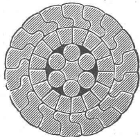
Patentiert „verschlossene“ Drahtseile.
