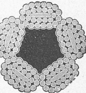
Patentiert „flachtzige“ Drahtseile.
