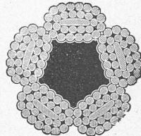
Patentirte „flachtzige“ Drahtseile.
