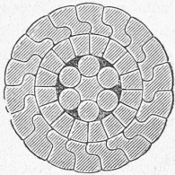
Patentiert „verschlossene“ Drahtseile.
