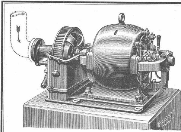
Hochdruckturbine mit direkt gekuppelter Gleichstromdynamo.
