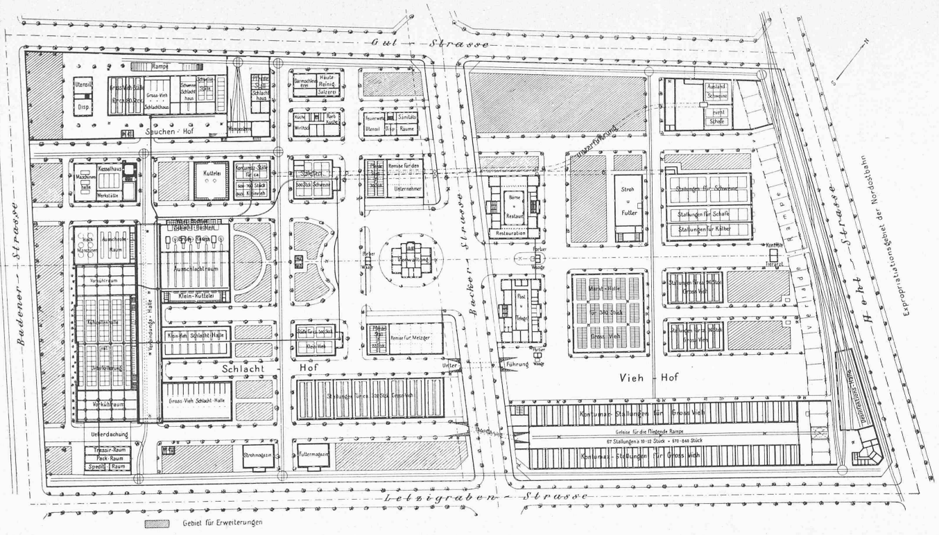
Das Schlacht- und Viehhofprojekt der Stadt Zürich. — Uebersichtsplan.
