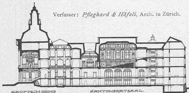
Schnitt C-D 1:1000.
