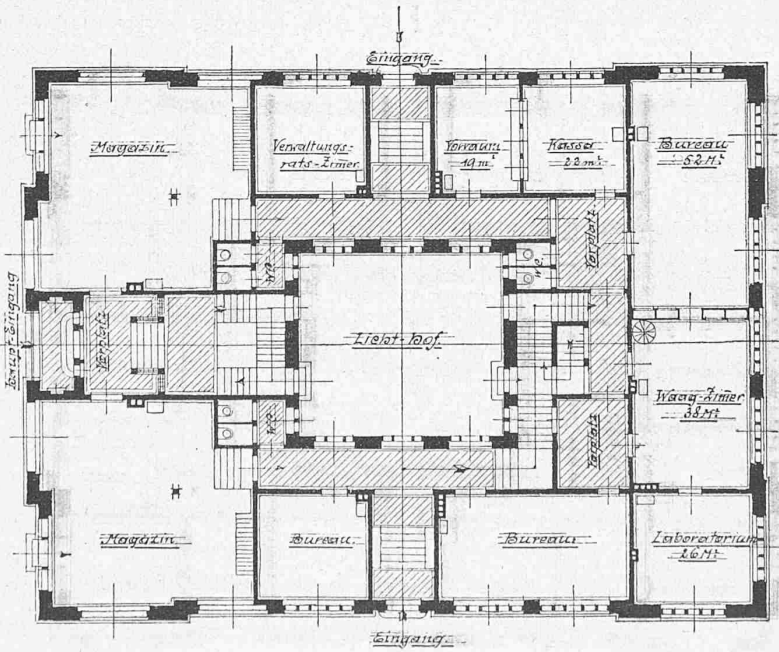
Erdgeschoss-Grundriss. — Masstab 1 : 300.
