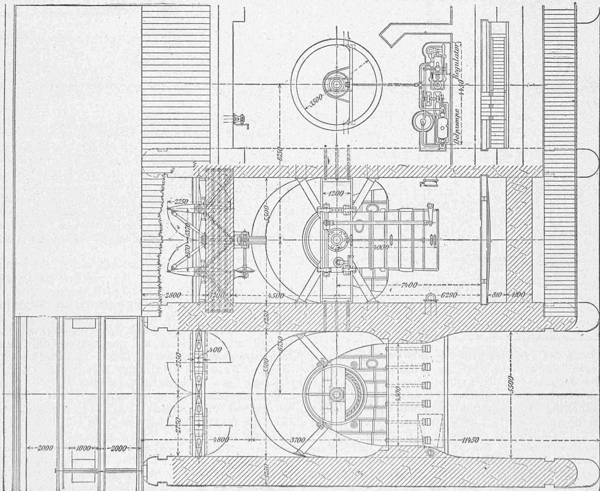
Fig. 3. Grundrisse 1:150.
