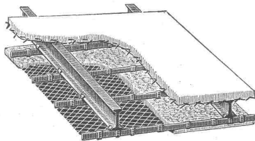
Deckenkonstruktion Hurdislatten und Gipslatten.
