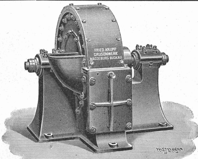
Schlagkreuzmühle.
