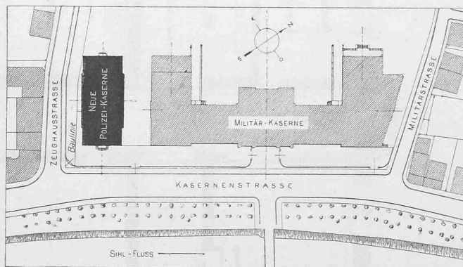
Lageplan. — Masstab 1 : 2500.
