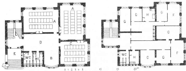
Grundriss vom Erdgeschoss. — 1 : 600. — Grundriss vom II. Obergeschoss.
