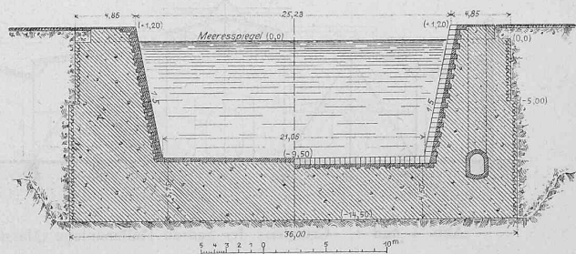
Abb. 8. Querschnitte der Eintrittskammer des Docks Nr. 1. — 1 : 500.
