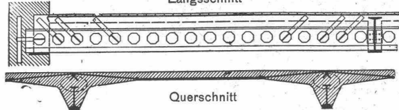
Längsschnitt
