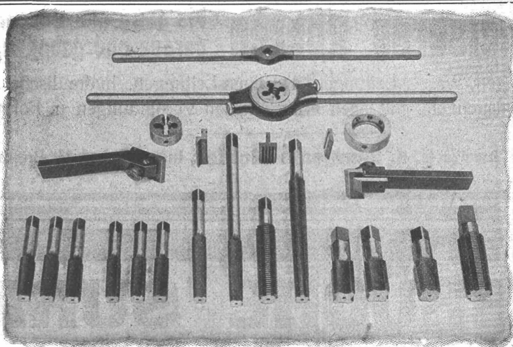
Gruppe von Gewindefräse-Werkzeugen.
