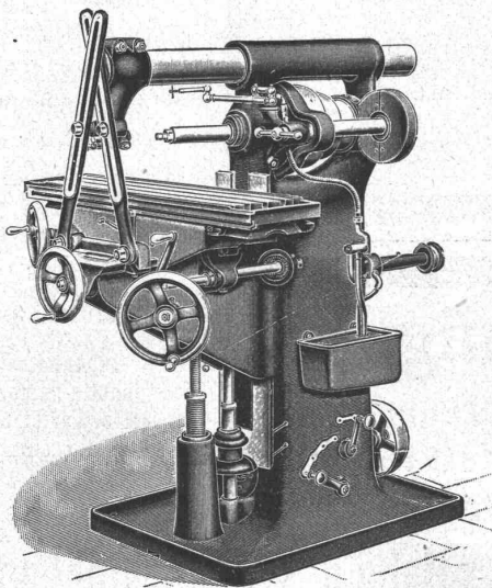
Einfahe Fräsmaschine. No. 2.
