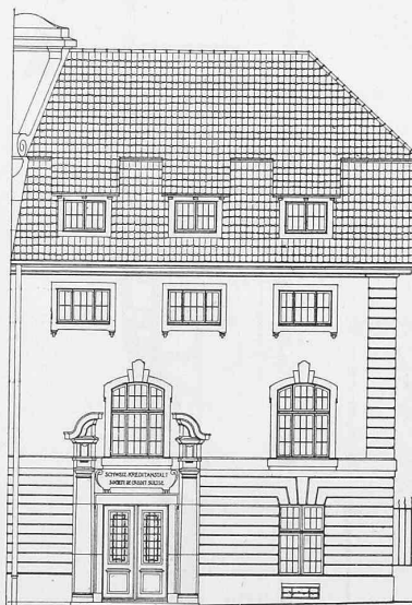
Abb. 9. Geometrische Ansicht der Fassade am Luftgässlein. — 1 : 200.
